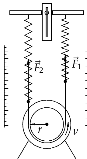
Slika 2: Pronyjeva zavora.
