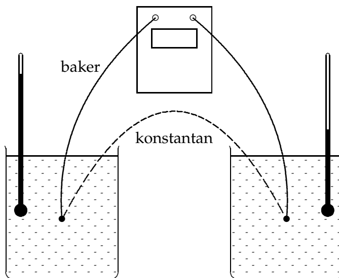
Slika 4: Umeritev termočlena
