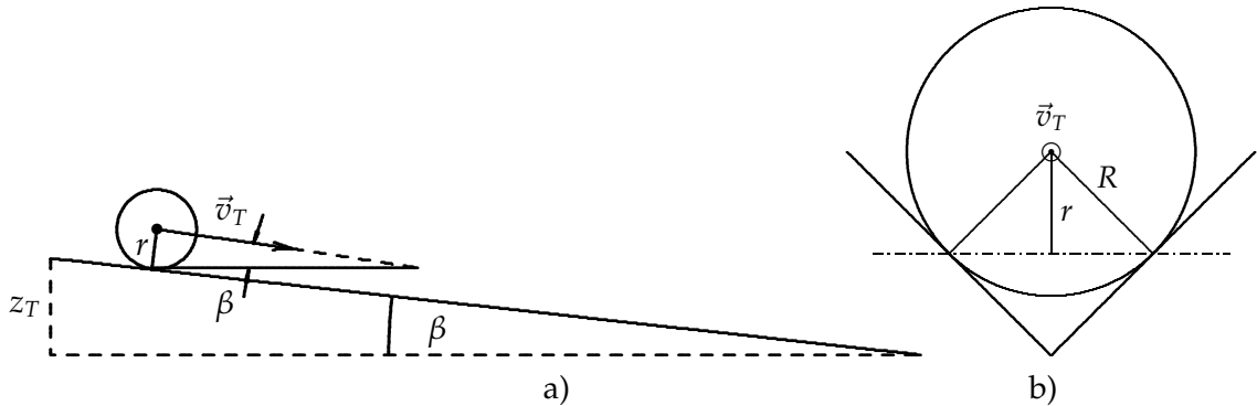
Slika 1: a) Kotaleči se valj na klancu in b) kroglica v žlebu, pogled od spredaj.
