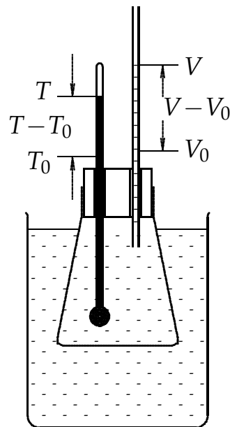
Slika 3: Merjenje razteznosti kapljevina.
